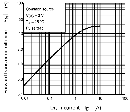
Fig. 8.8 |Y_{fs}| - I_D
